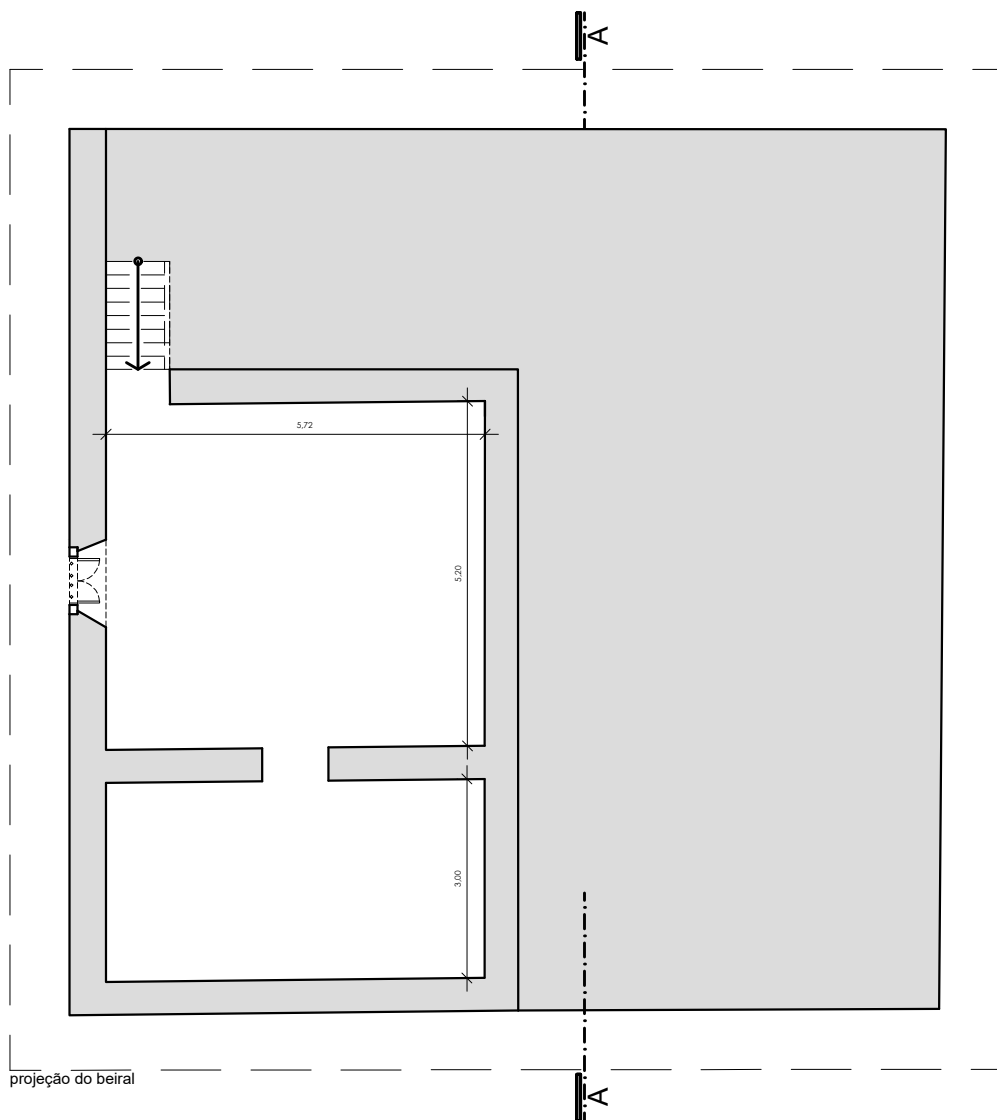
PLANTA SOBRADO
