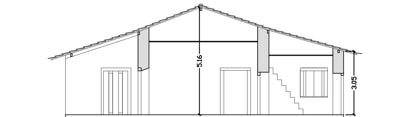
CORTE AA
