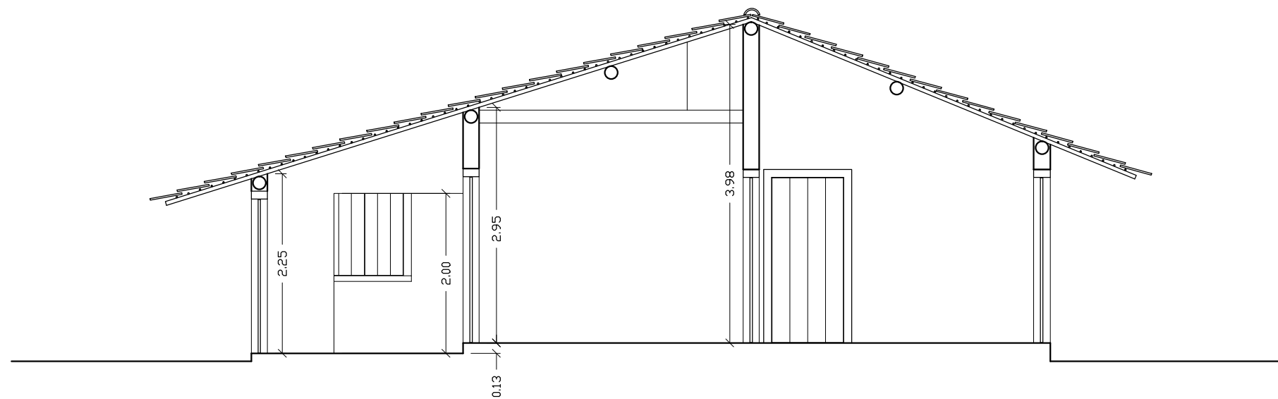
CORTE BB
