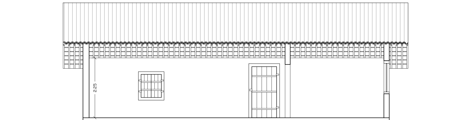
CORTE AA
