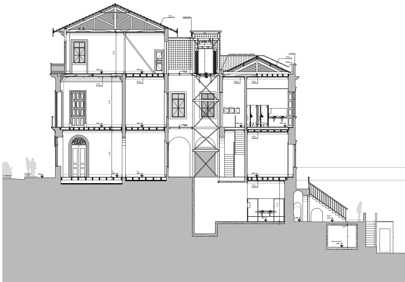
CORTE AA
