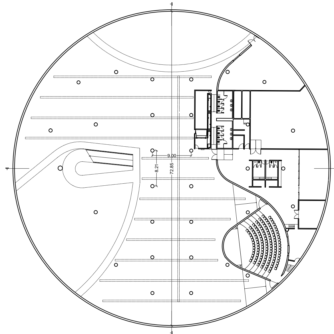
PLANTA SUBSOLO
