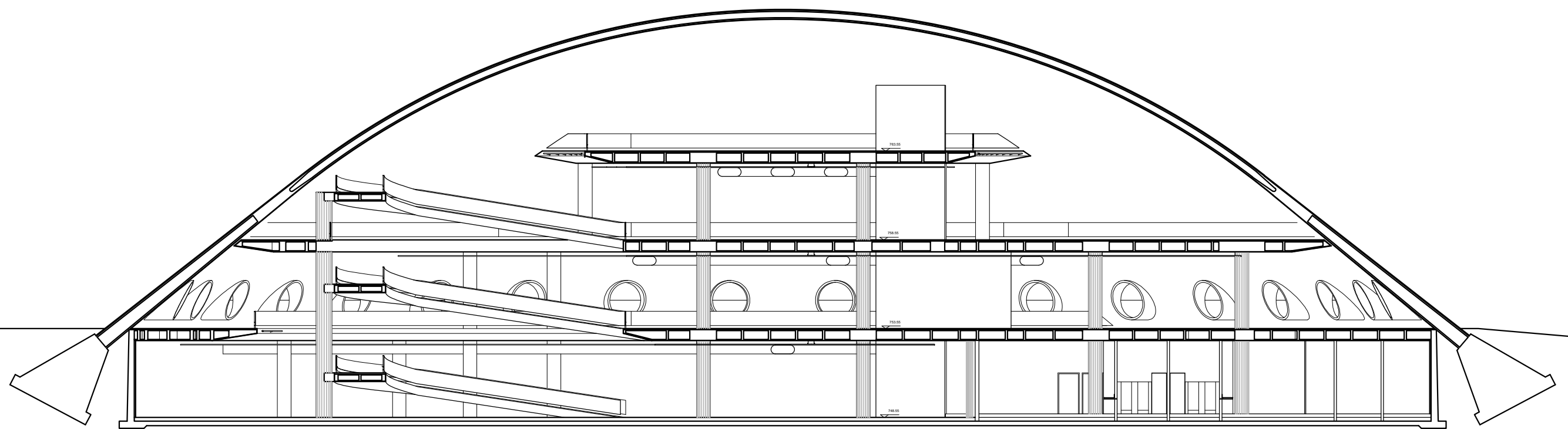
CORTE BB
