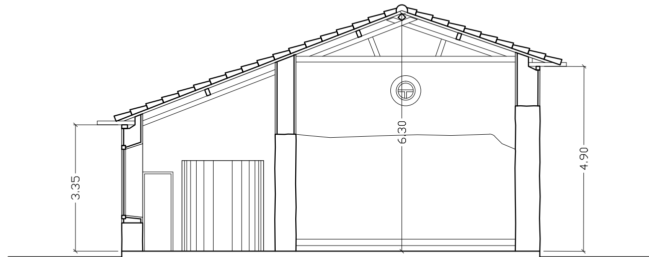
CORTE CC
